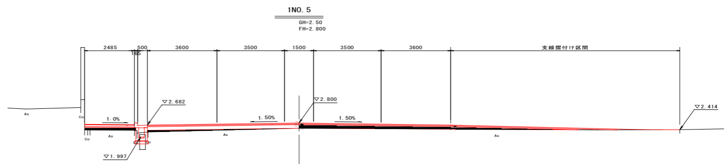
2工区標準断面
