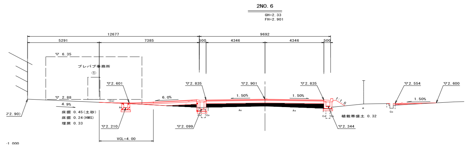
2工区標準断面
